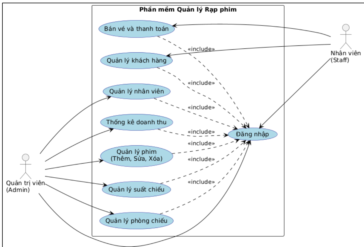
Hình 2.1. Sơ đồ UseCase tổng quát
